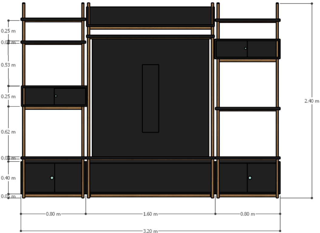
Alzado
